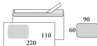
E65 isolla ikkunalla, kontakti isoikkunakuori, silikonipeitetarra pitkällä sivulla
