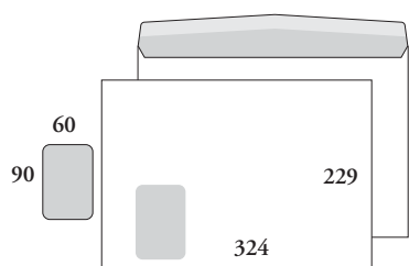
C4 isolla ikkunalla isoikkunakuori, kostutettava liima pitkällä sivulla
