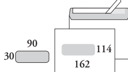
C6 ikkuna, kontakti ikkunakuori, silikonipeitetarra pitkällä sivulla
